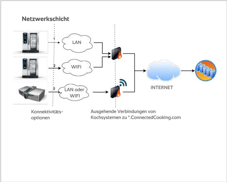
Abb. 1: Netzwerkschicht
