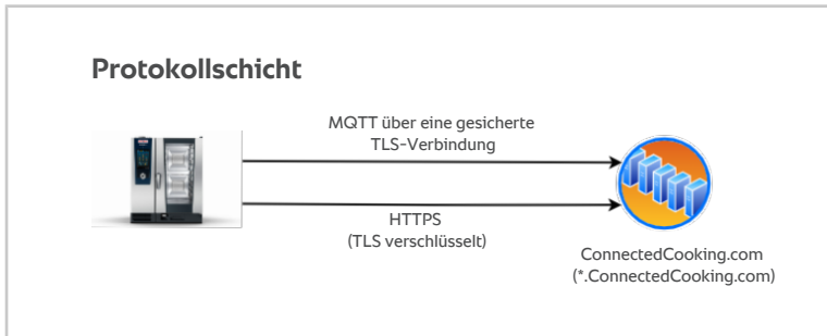
Abb. 2: Protokollschicht
